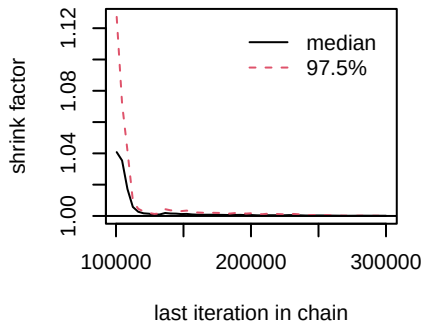
d.I.Rociletinib
